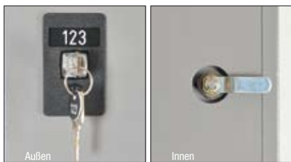
L/F Zylinderschloss (Plättchenzylinder) mit 2 Eigenschlüsseln
