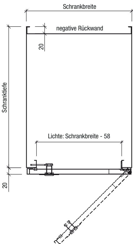
Perfortür aufschlagend mit Perforationsstanzung Quadrat 10 mm, Steg 5 mm oben und unten
